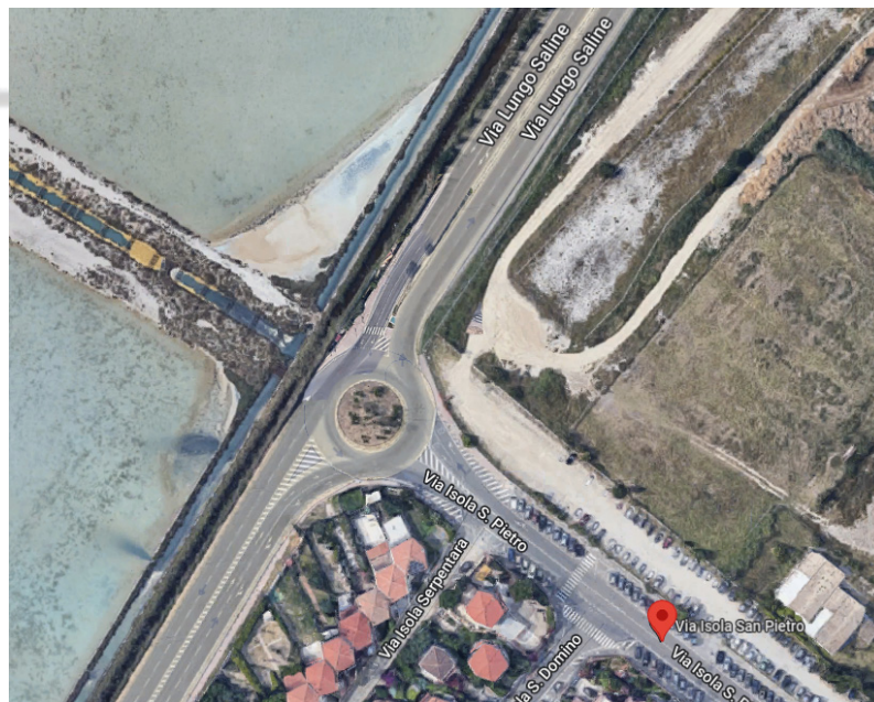
ROTATORIA VIA ISOLA SAN PIETRO/LUNGOSALINE - PROPOSTA
