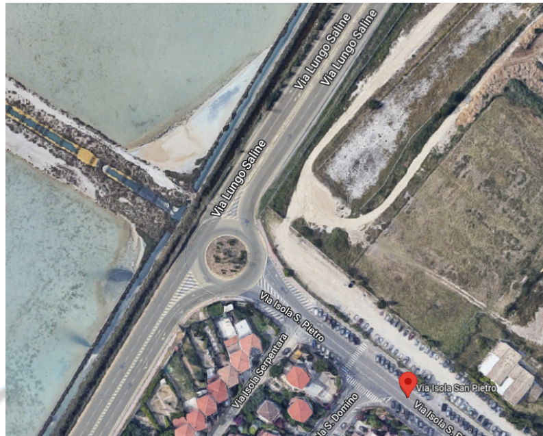
ROTATORIA VIA ISOLA SAN PIETRO/LUNGOSALINE - ATTUALE
